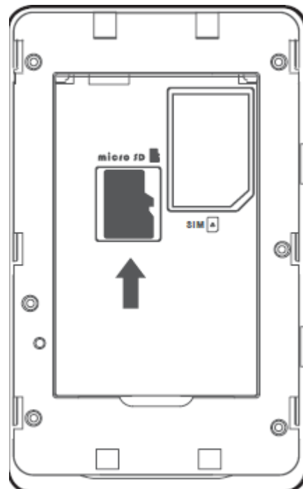
Gắn thẻ nhớ microSD vào khe thẻ nhớ
